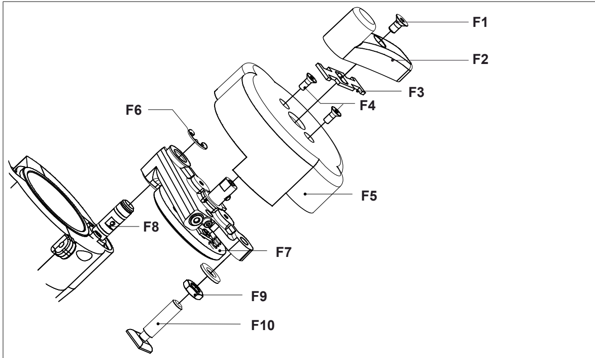
Bild 6.7/1: Austausch der Verschußbaugruppe
