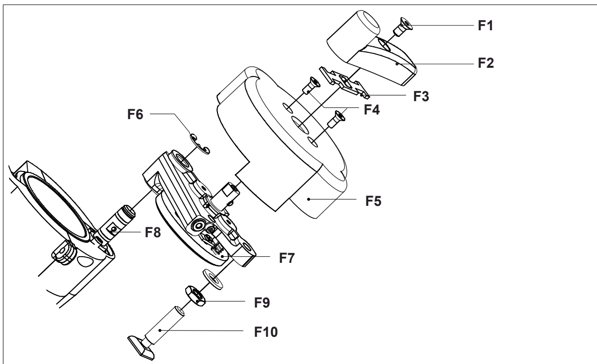
Afbeelding 6.7/1: Uitwisseling van de afsluitmodule
