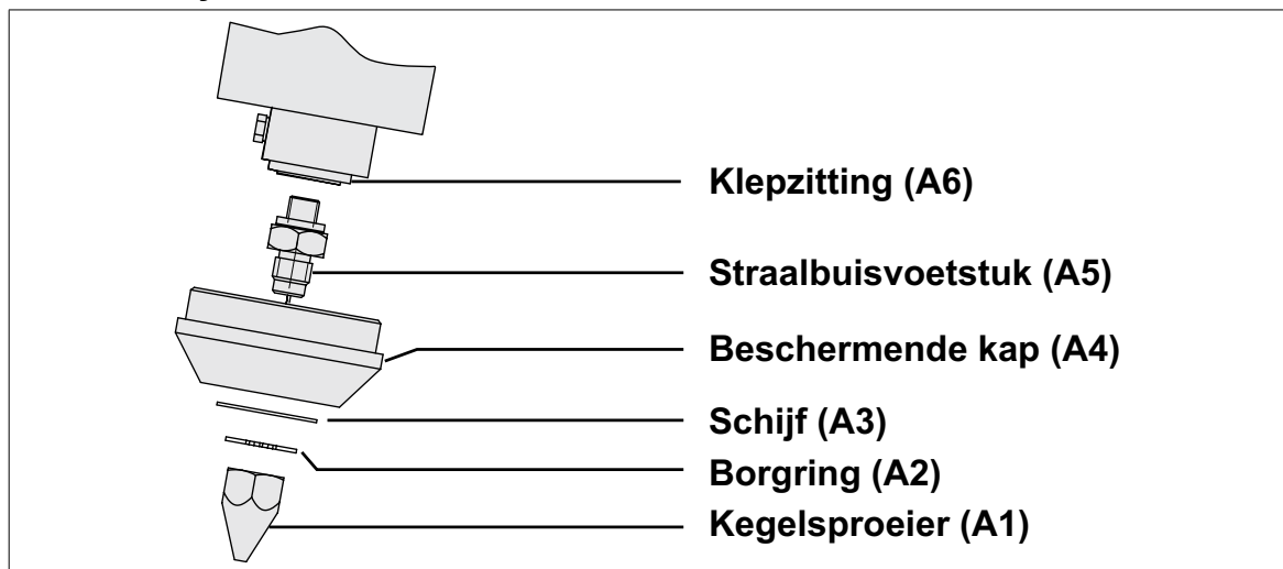
Afbeelding 6.3/1: Straalbuissysteem in detail
