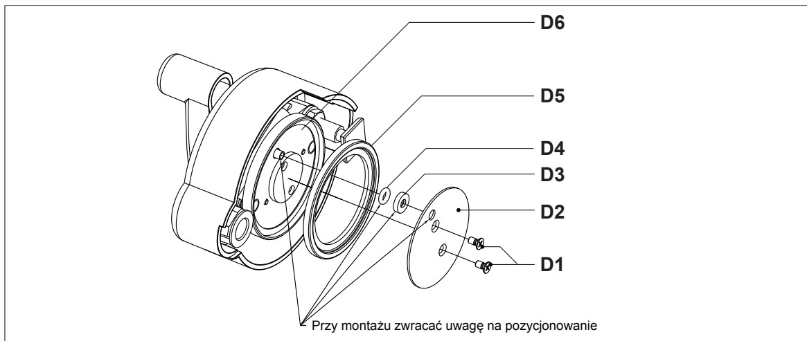
Rys. 6.5/1: Wymiana uszczelki z pokrywy zbiornika pistoletu
