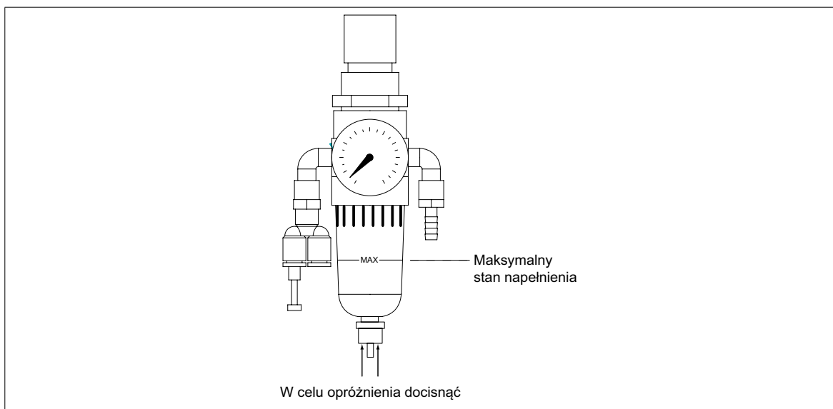
Rys. 6.1/1: Opróżnianie oddzielną wody
