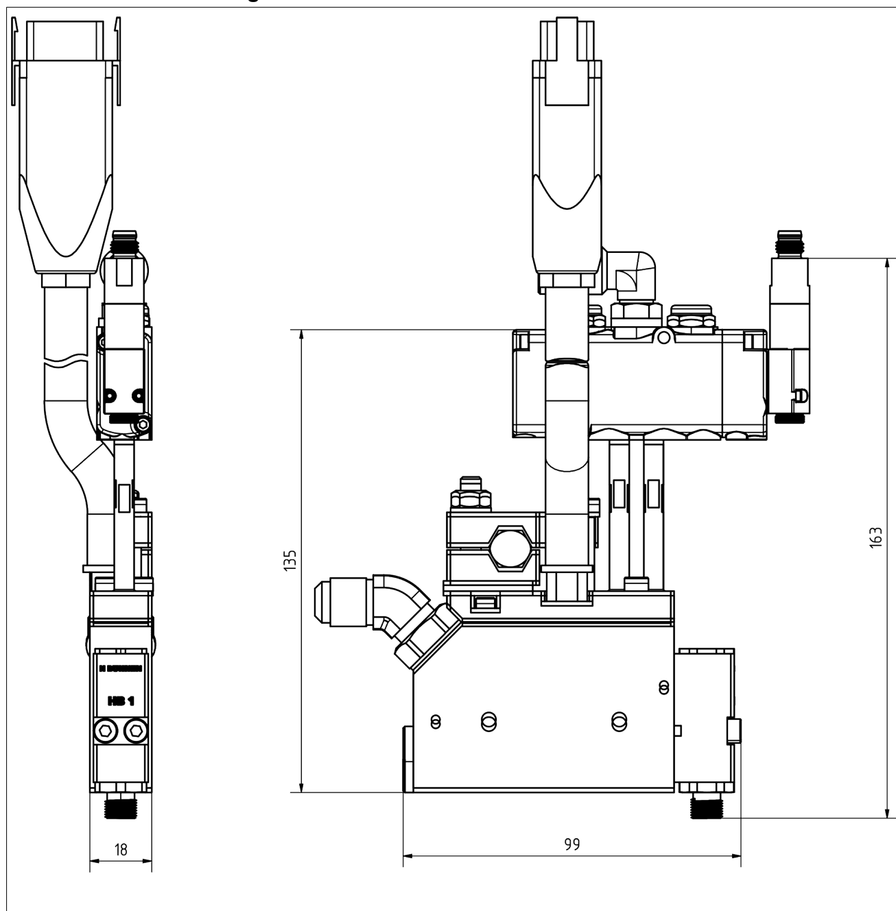
Bild 1: Maßzeichnung
