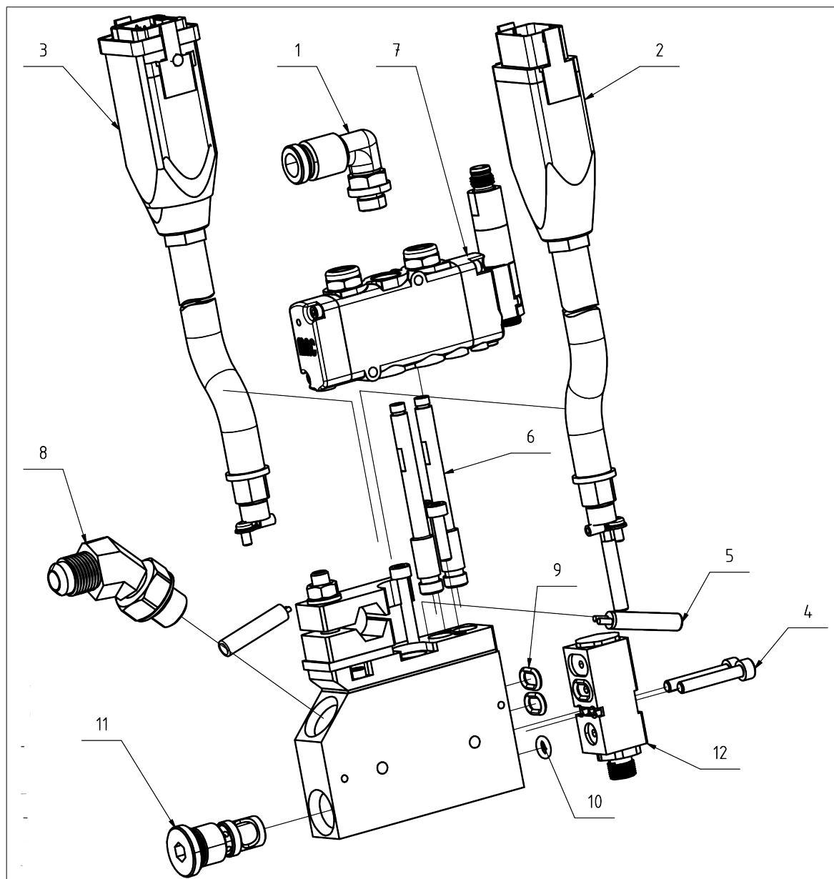
Bild 5: Ersatzteile
